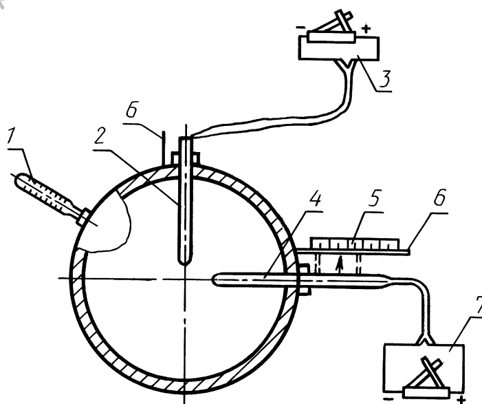
Схема установки приборов в газоходе
