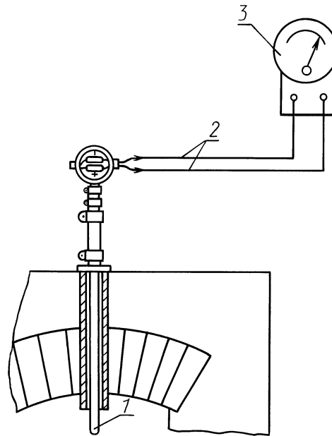
Схема установки термопары
