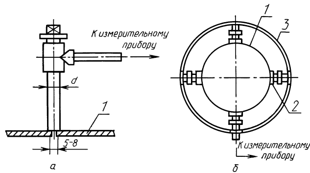
1 — стенка газохода; 2 — патрубок; 3 — соединительный трубопровод
